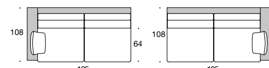
BW-122-3021 Abschlusselement 2/92,5 tief re/li
