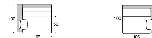
Gesamtbreite: TYP 1 – 123 TYP 2 – 133 TYP 3 – 123 TYP 4 – 123 TYP 5 – 123 TYP 6 – 123
