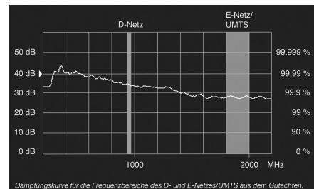
Dämpfungskurve für die Frequenzbereiche des D- und E-Netzes/UMTS aus dem Gutachten.
