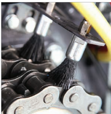
Kettenschmierung
