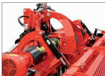
Hydraulische Walzenverstellung
