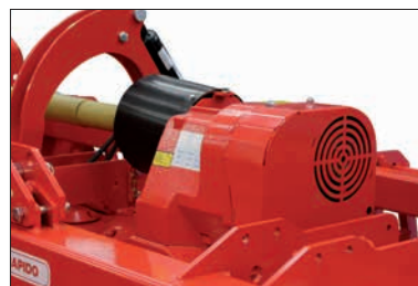
Luftkühlung Seitengetriebe
