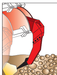
Hydropneumatische Steinsicherung
