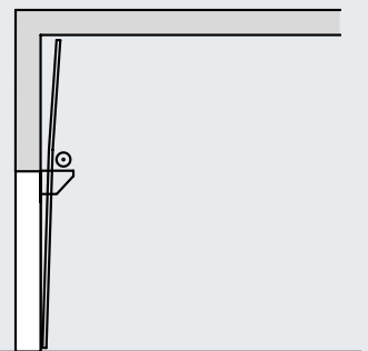
Beschlag VU mit unten liegender Federwelle
