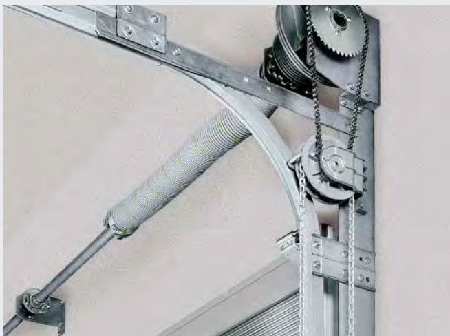
Optional: Handkettenzug
