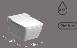
Tiefspül-WC B 350 / T 540 spülrandlos, 4,5/6l, wandhängend → WC-Sitz mit Absenkautomatik
