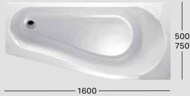
Badewanne L 1600 / B 500 / 750 / T 420 mit Raumspareffekt, links
