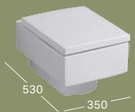
Tiefspül-WC B 350 / T 530 6l, wandhängend → WC-Sitz mit Absenkautomatik
