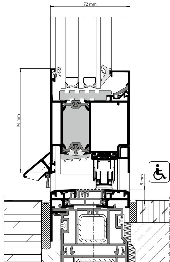
heroal D 72, Schnittdarstellung barrierefrei nach DIN 18040
