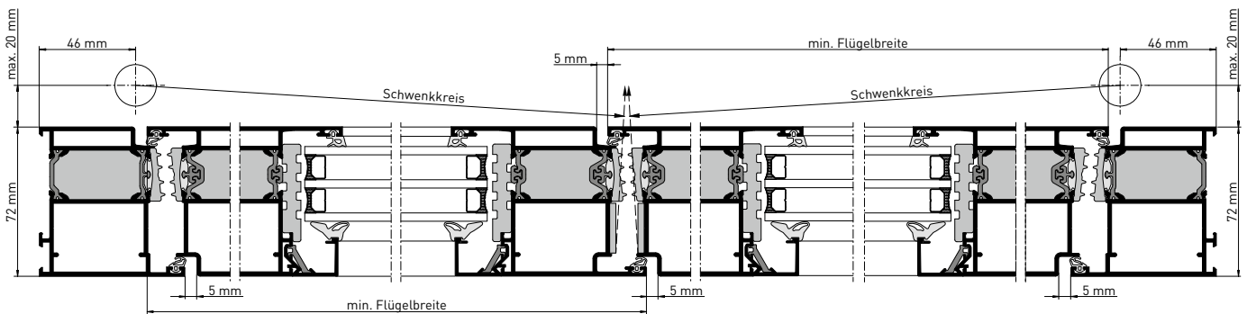
heroal D 72, Schnittdarstellung Fähigkeit zur Freigabe, Spaltmaß 5 mm
