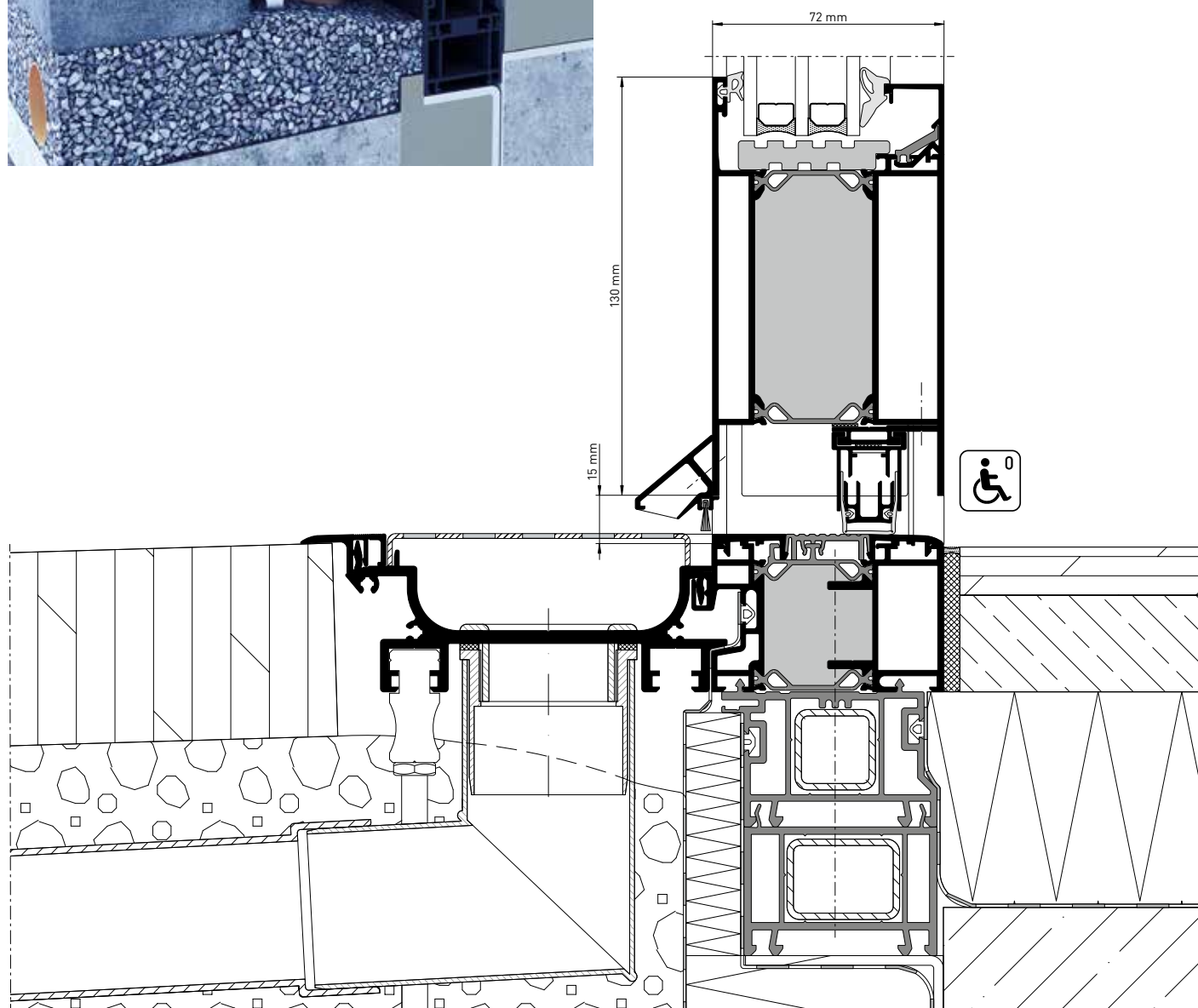
heroal D 72, Schnittdarstellung Null-Barriere nach DIN 18040
