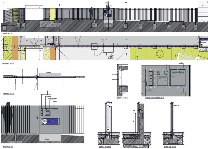
Detailplan Zaunanlage
