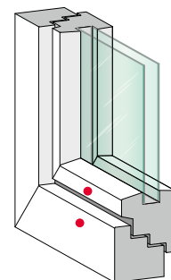
halbflächenversetzt
