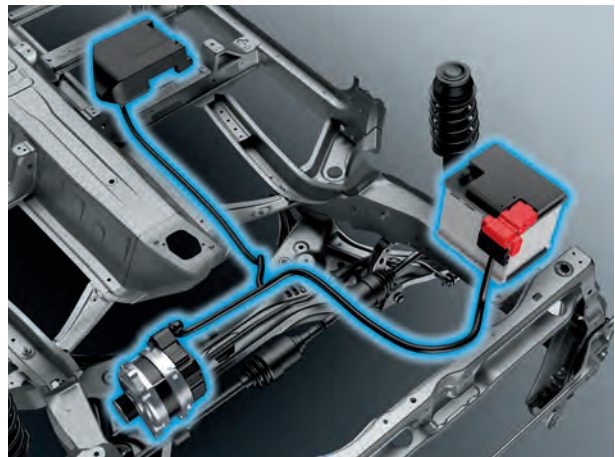
ISG und Lithium-Ionen-Batterie sind die Bestandteile des SHVS Mild Hybrid Systems
