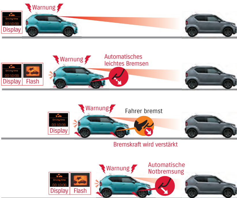
Dual-Camera gestützte aktive Bremsunterstützung (DCBS) 1,2
