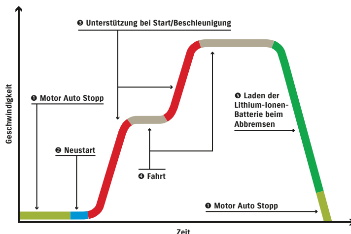
Funktionsweise des SHVS Mild Hybrid Systems
