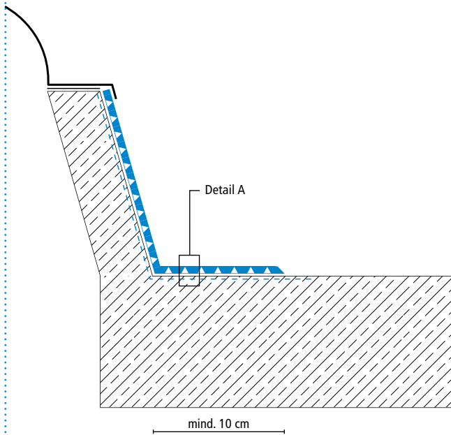
Zeichnung Nr.: ProThan Detail-3503
