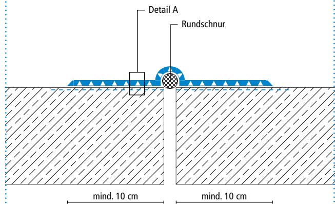
Zeichnung Nr.: ProThan Detail-3507
