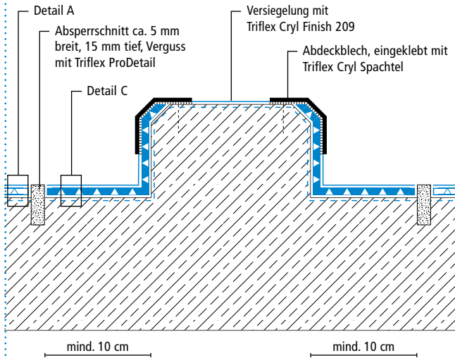
Zeichnung Nr.: DeckCoat-1704
