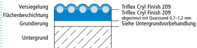
Systemaufbau – Detail A
