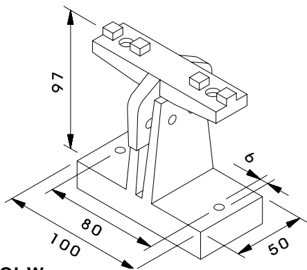
VARISOL W500 seitenverstellbare Montagekonsole, Verstellbereich 15mm nach rechts und links
