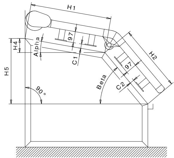
VARISOL W500 mit Eckumlenkung, Ausführung 2
