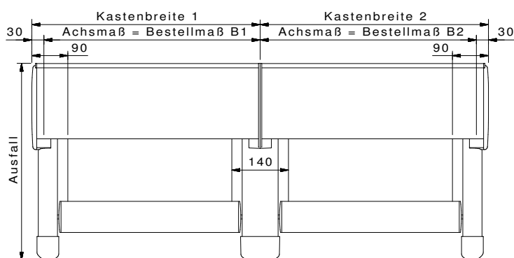
VARISOL W300 Draufsicht zweiteilig
