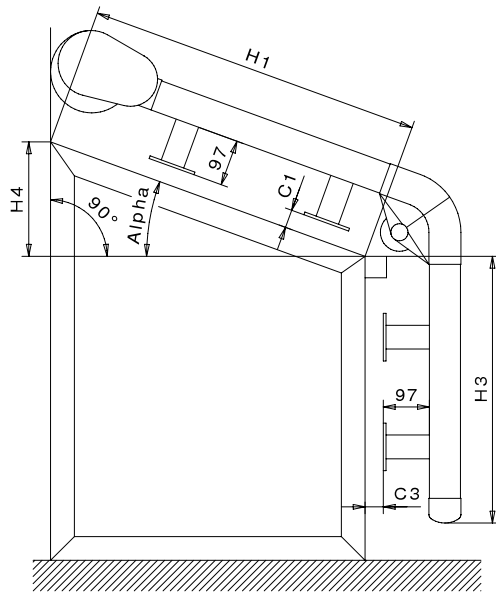
VARISOL W500 mit Eckumlenkung, Ausführung 1
