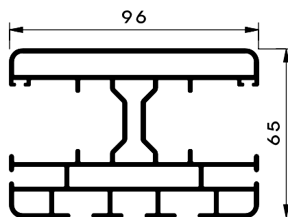
VARISOL W500 Mittelführungsschiene
