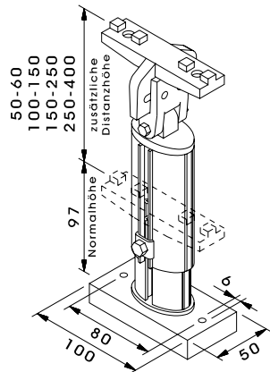
VARISOL W500 verlängerte Montagekonsole, höhenverstellbar
