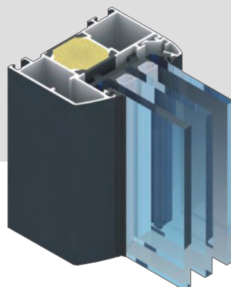
Seitenteilelement ISOGLAS U_g = 0,7 \text{ W/m}^2\text{K}
