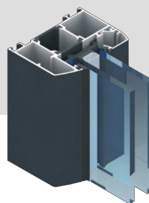
Seitenteilelement ISOGLAS U_g = 1,1 \text{ W/m}^2\text{K}
