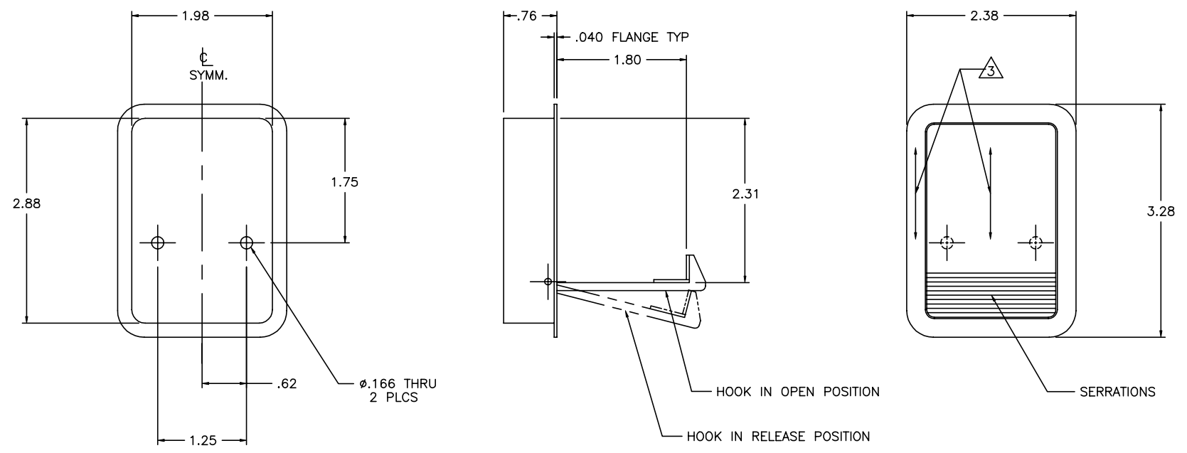
-1 DOOR RETAINER
